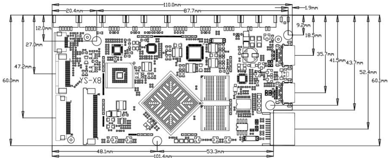
尺寸图
