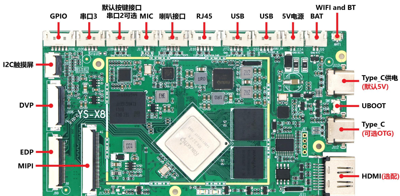
正面接口图
