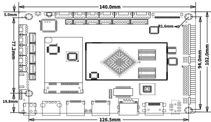
外形尺寸图
