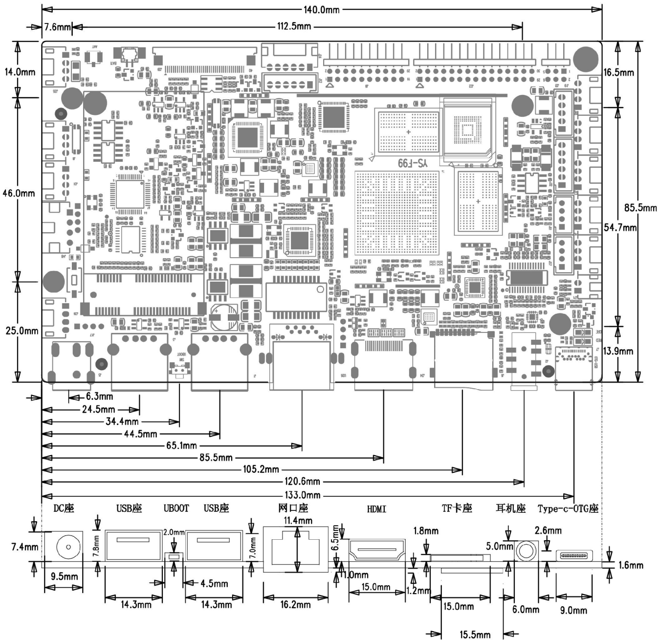
尺寸图
