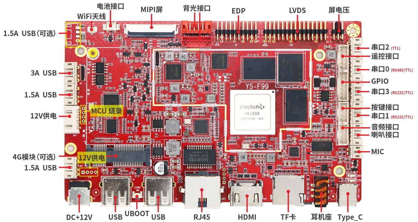
正面接口图
