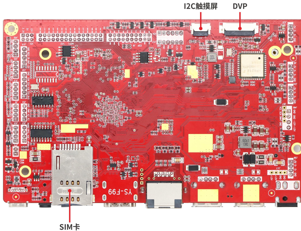
背面接口图
