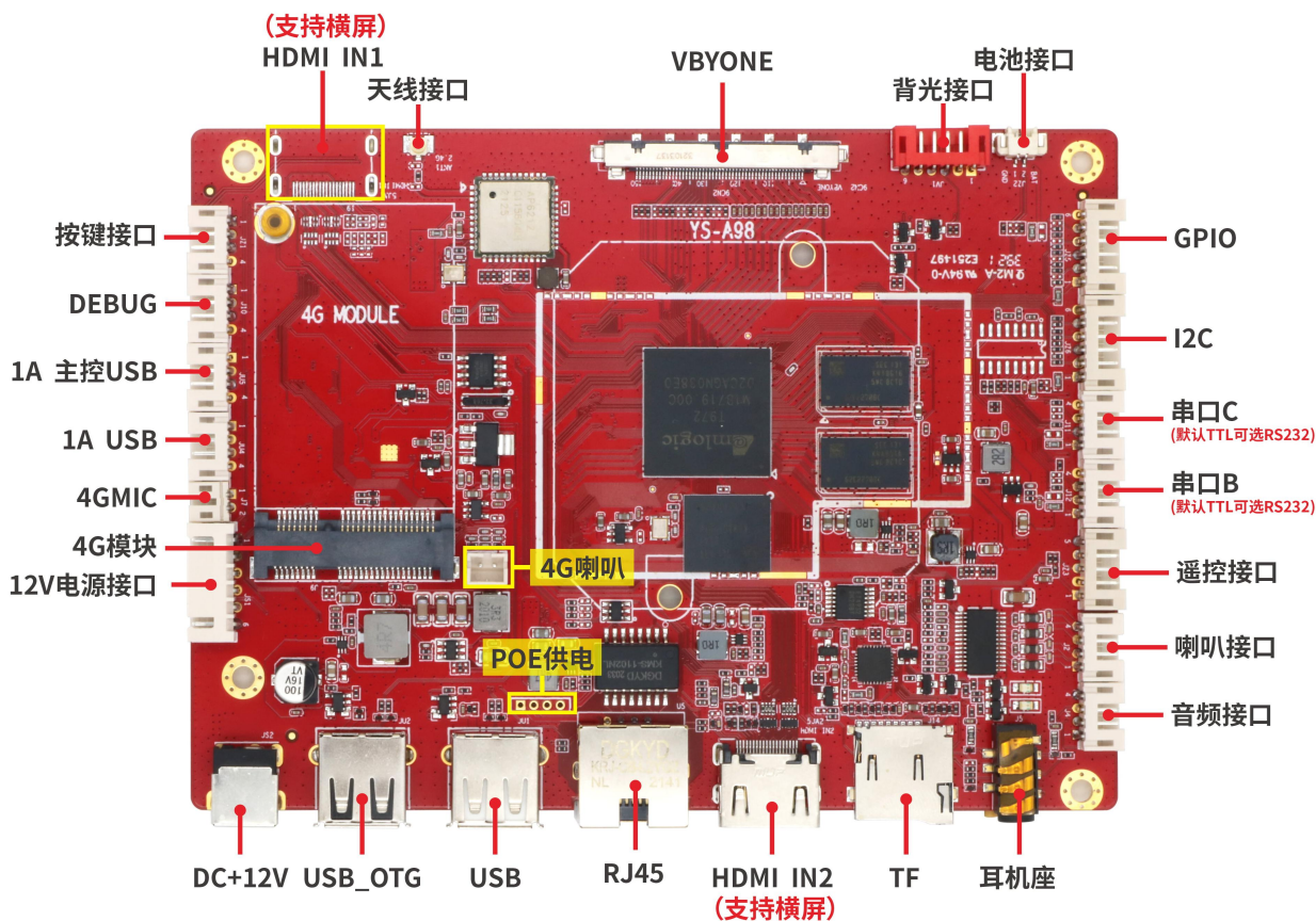
正面接口图
