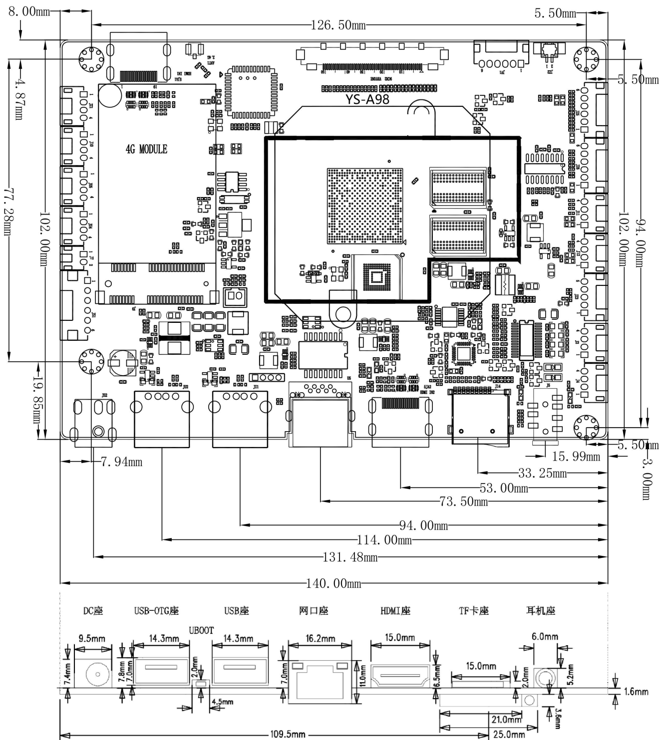
尺寸图
