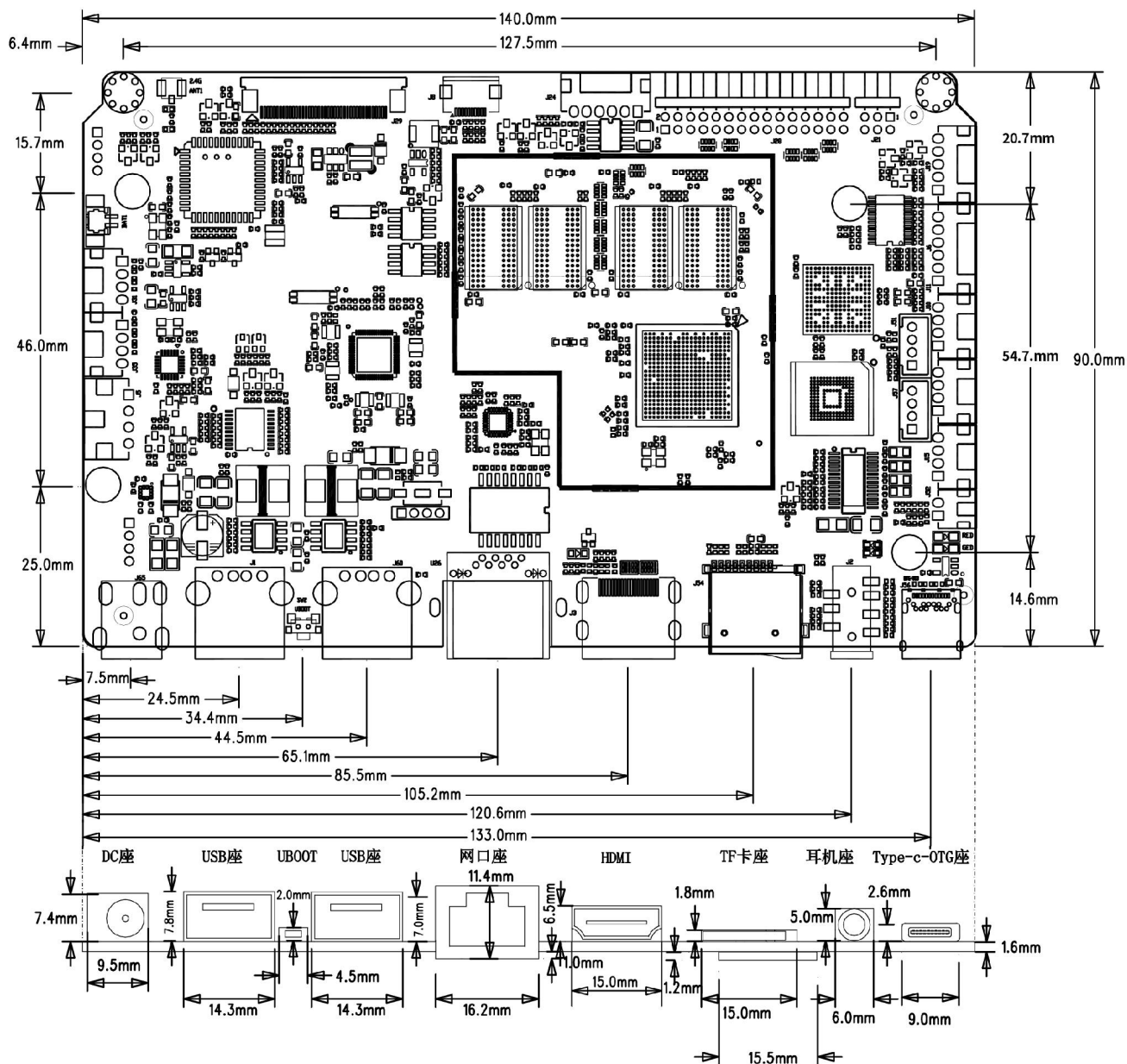
尺寸图
