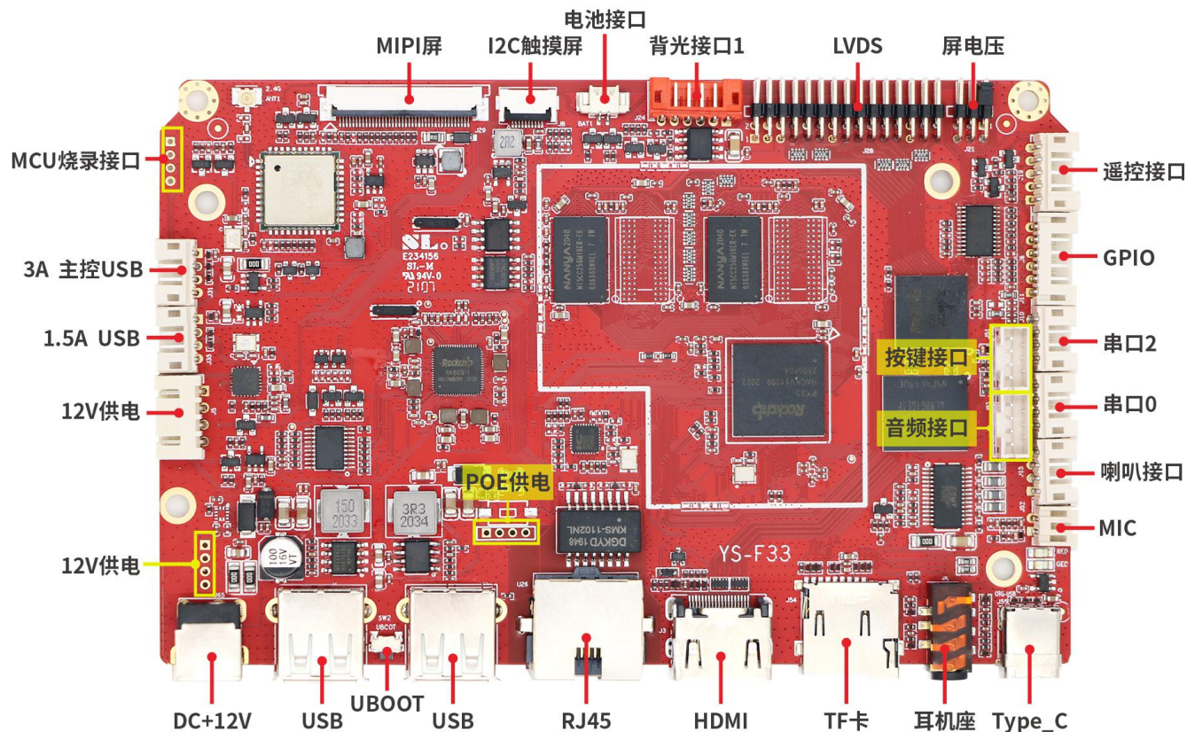
正面接口图
