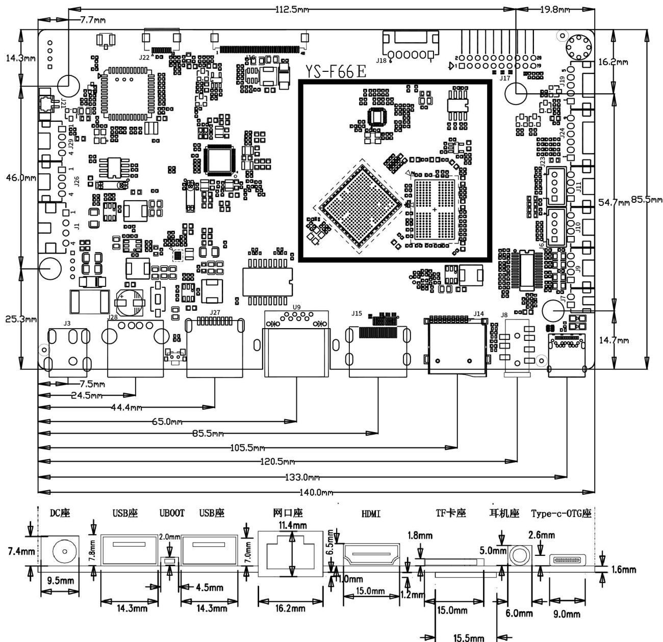
尺寸图
