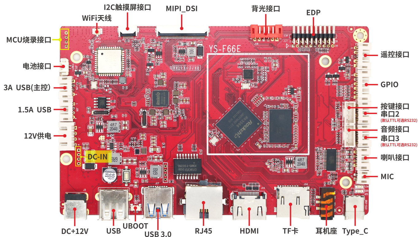
正面接口图
