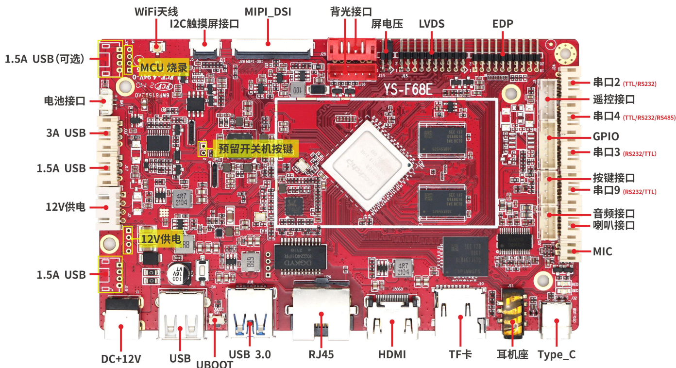
正面接口图
