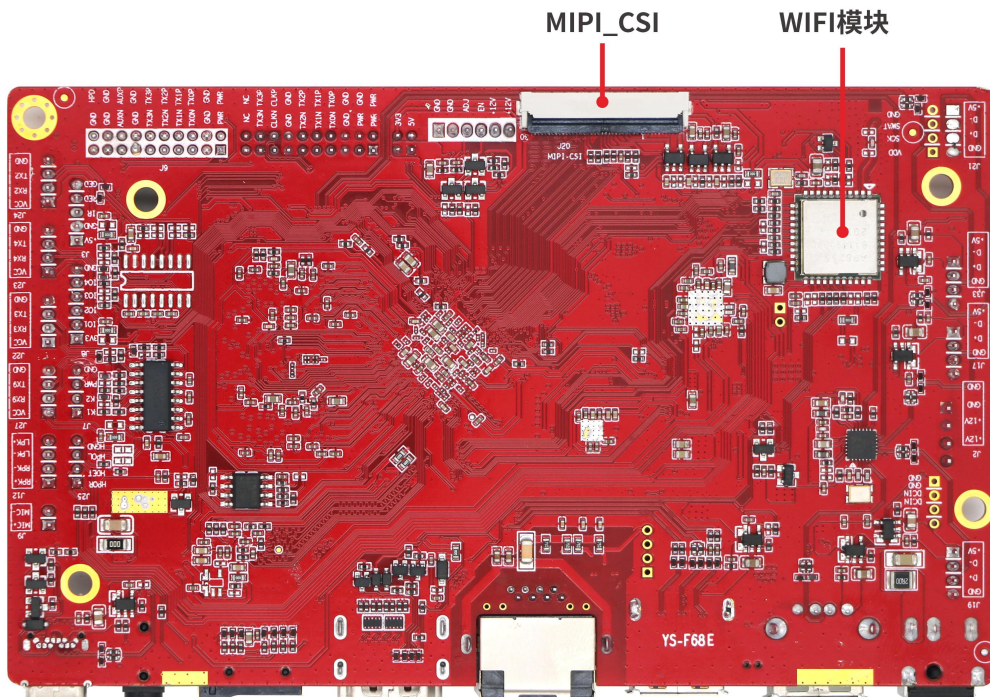
背面接口图
