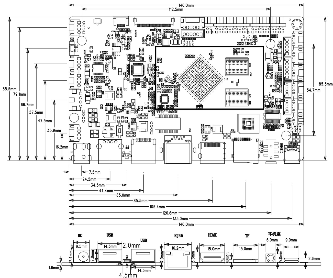
尺寸图
