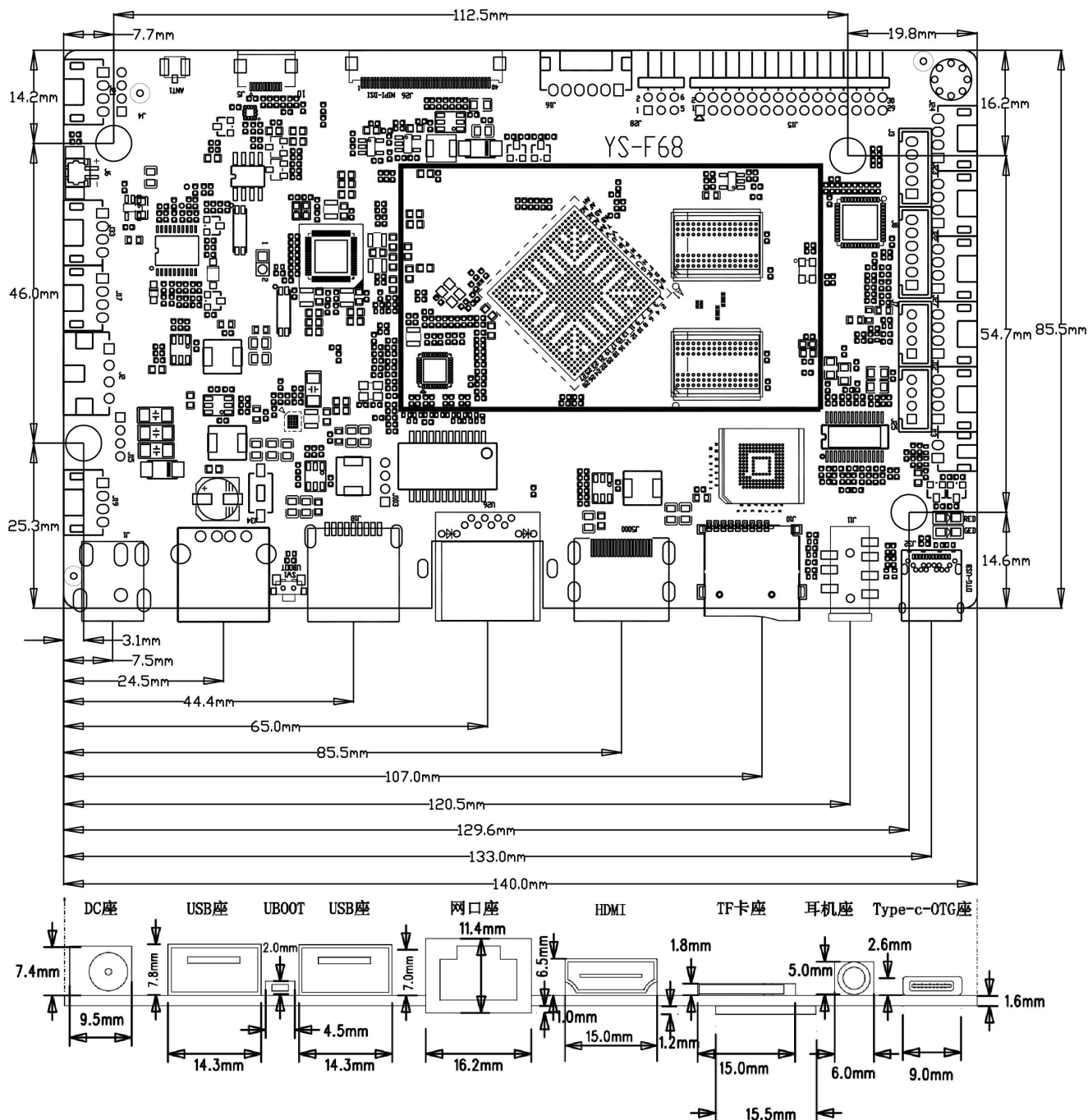
尺寸图
