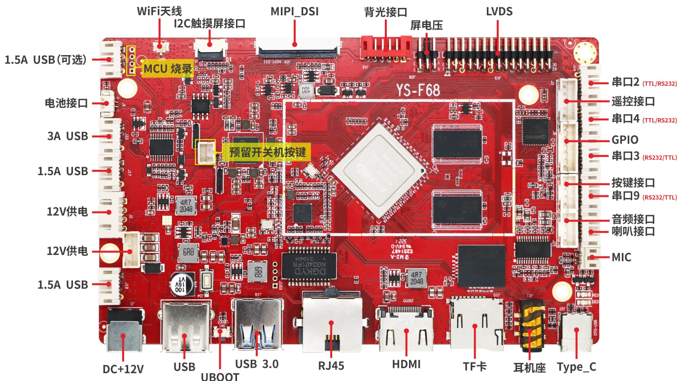
正面接口图
