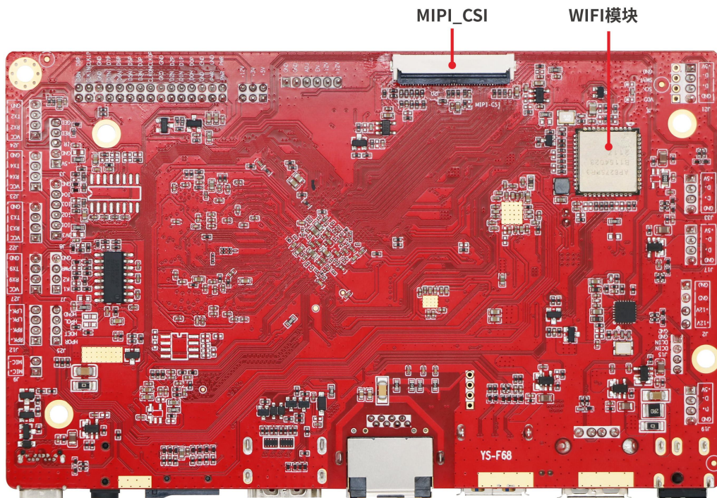
背面接口图
