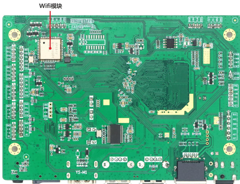
背面接口图
