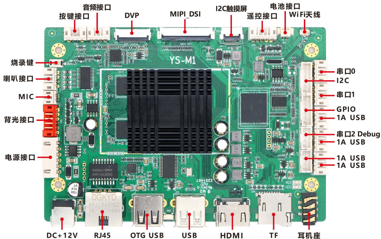
正面接口图
