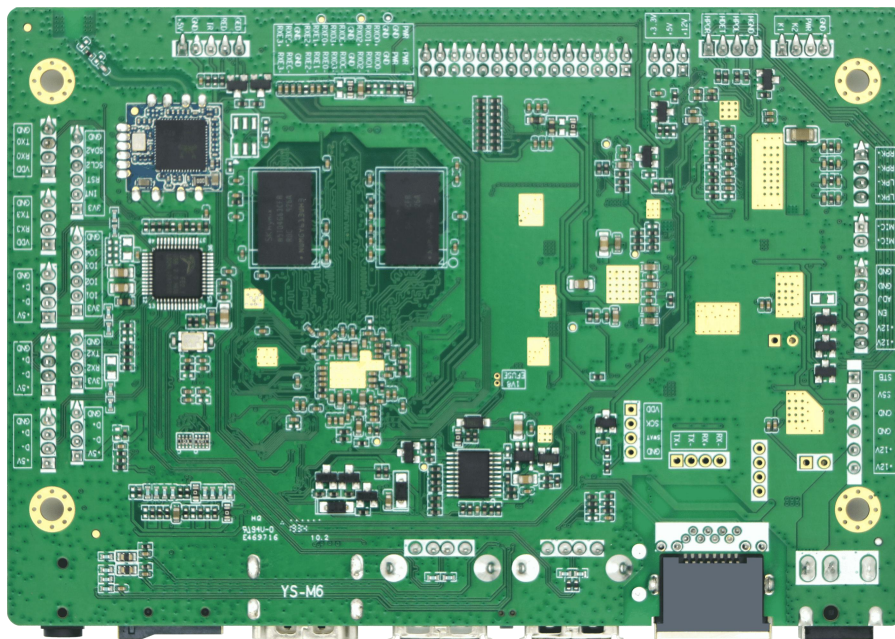
背面接口图
