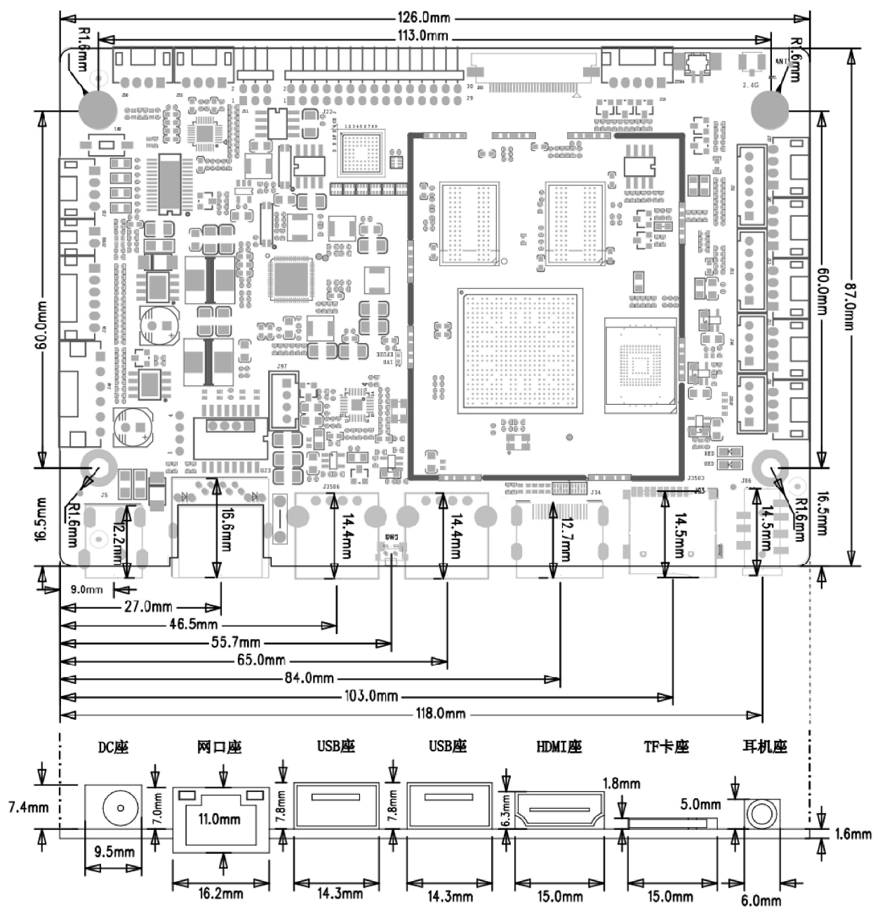
尺寸图
