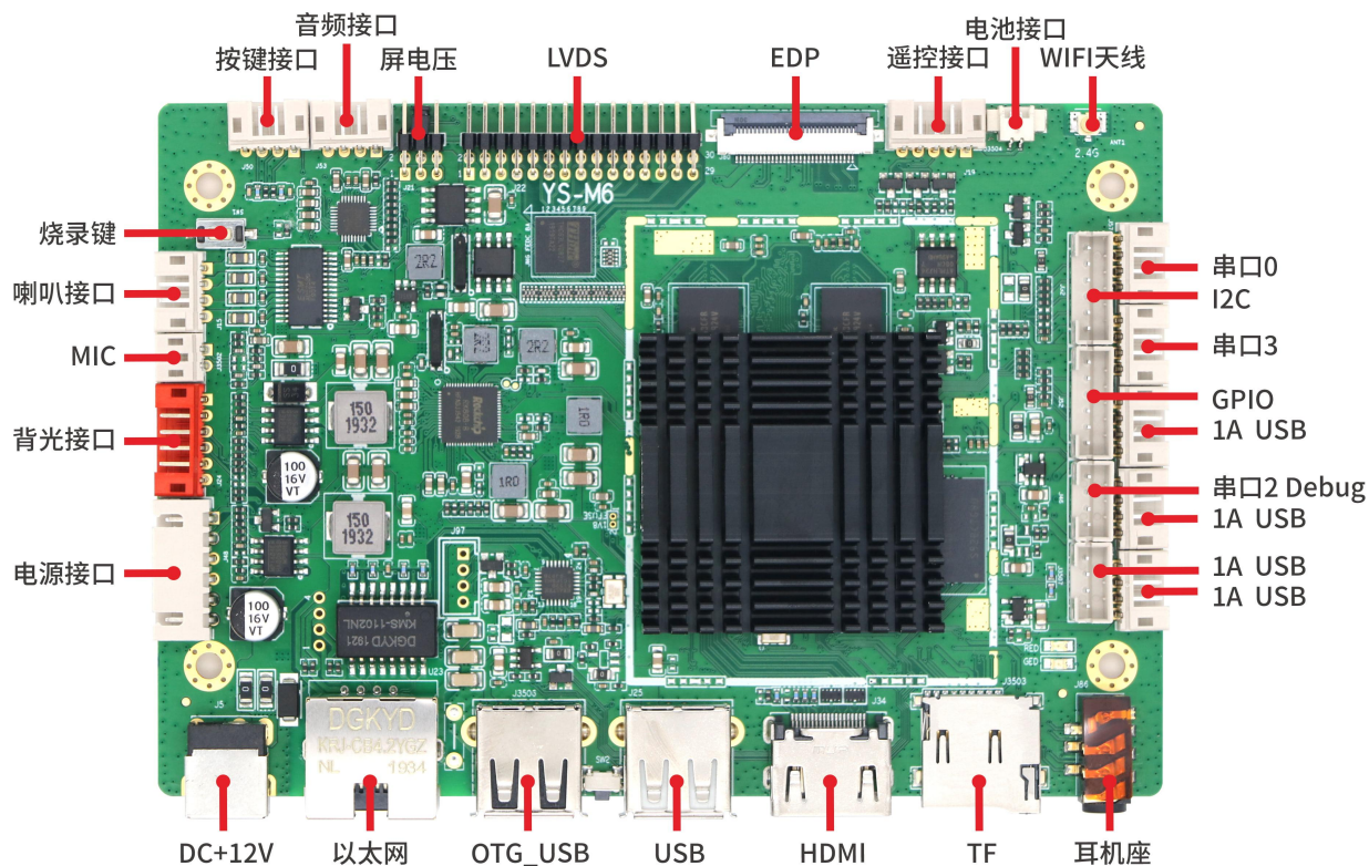
正面接口图
