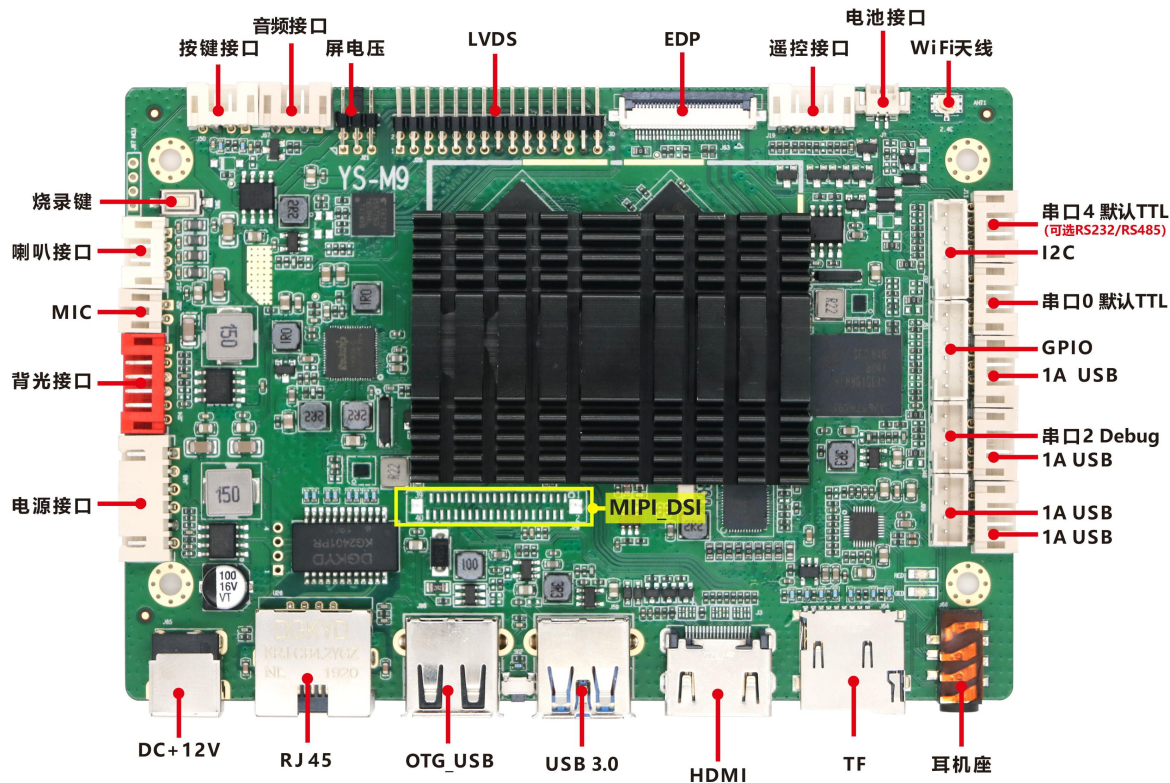
正面接口图
