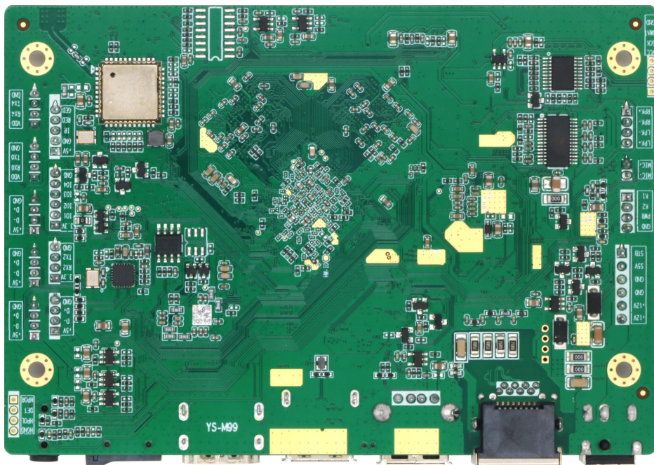
背面接口图
