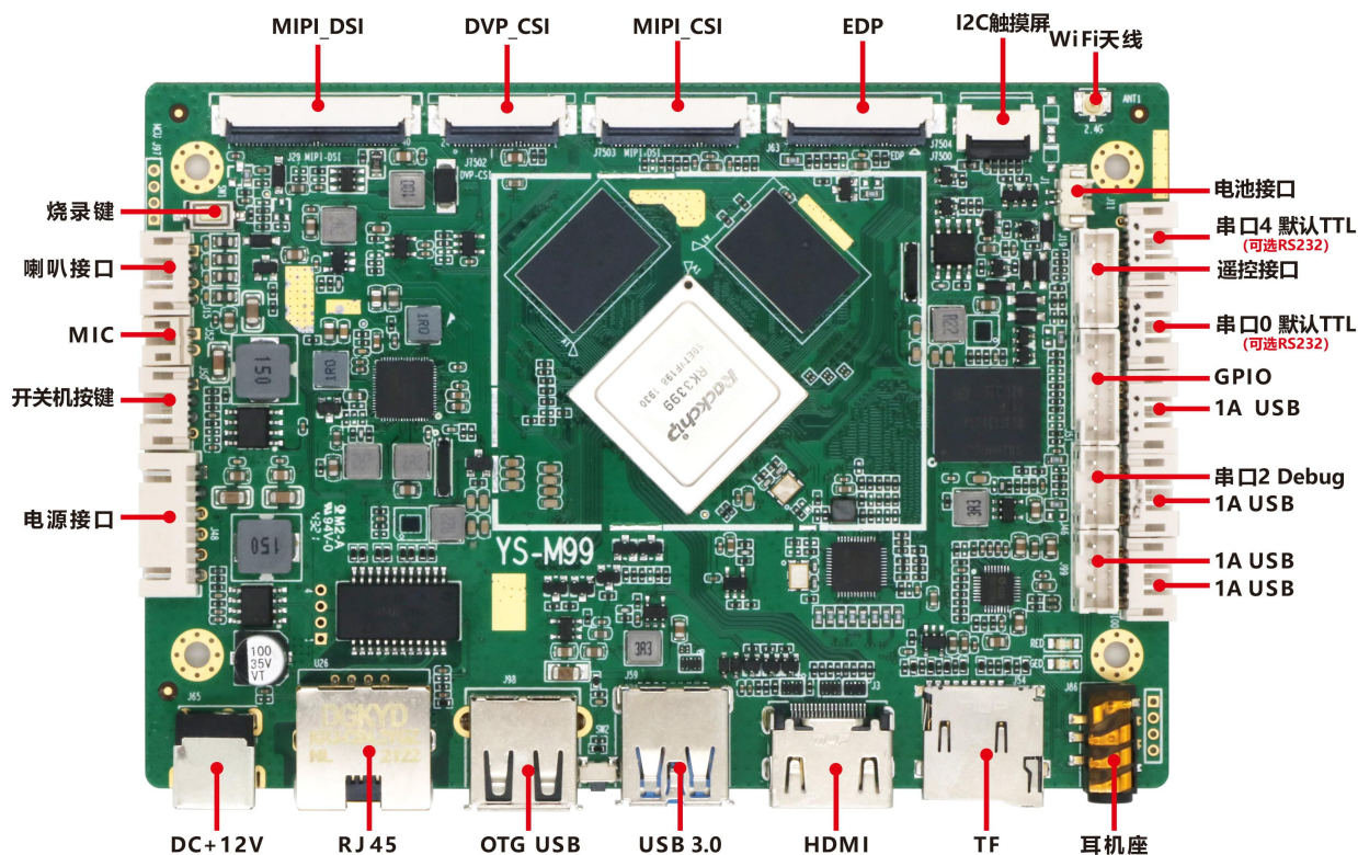
正面接口图
