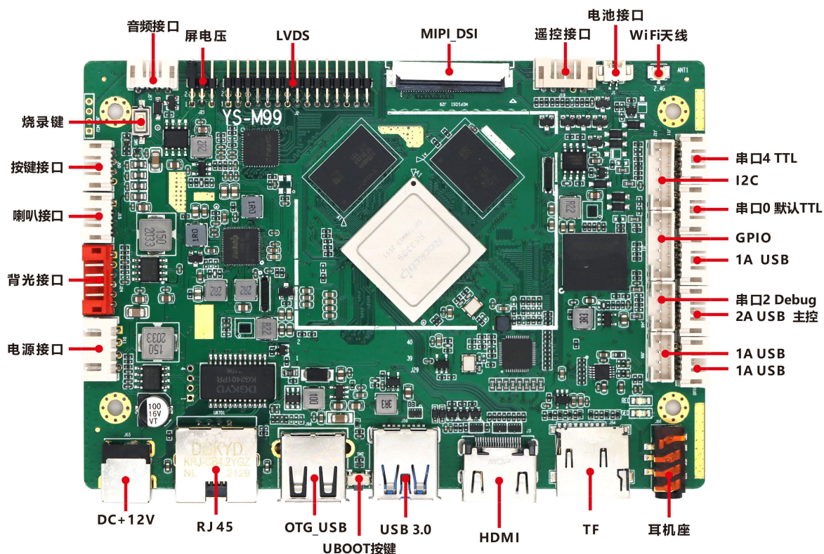
正面接口图
