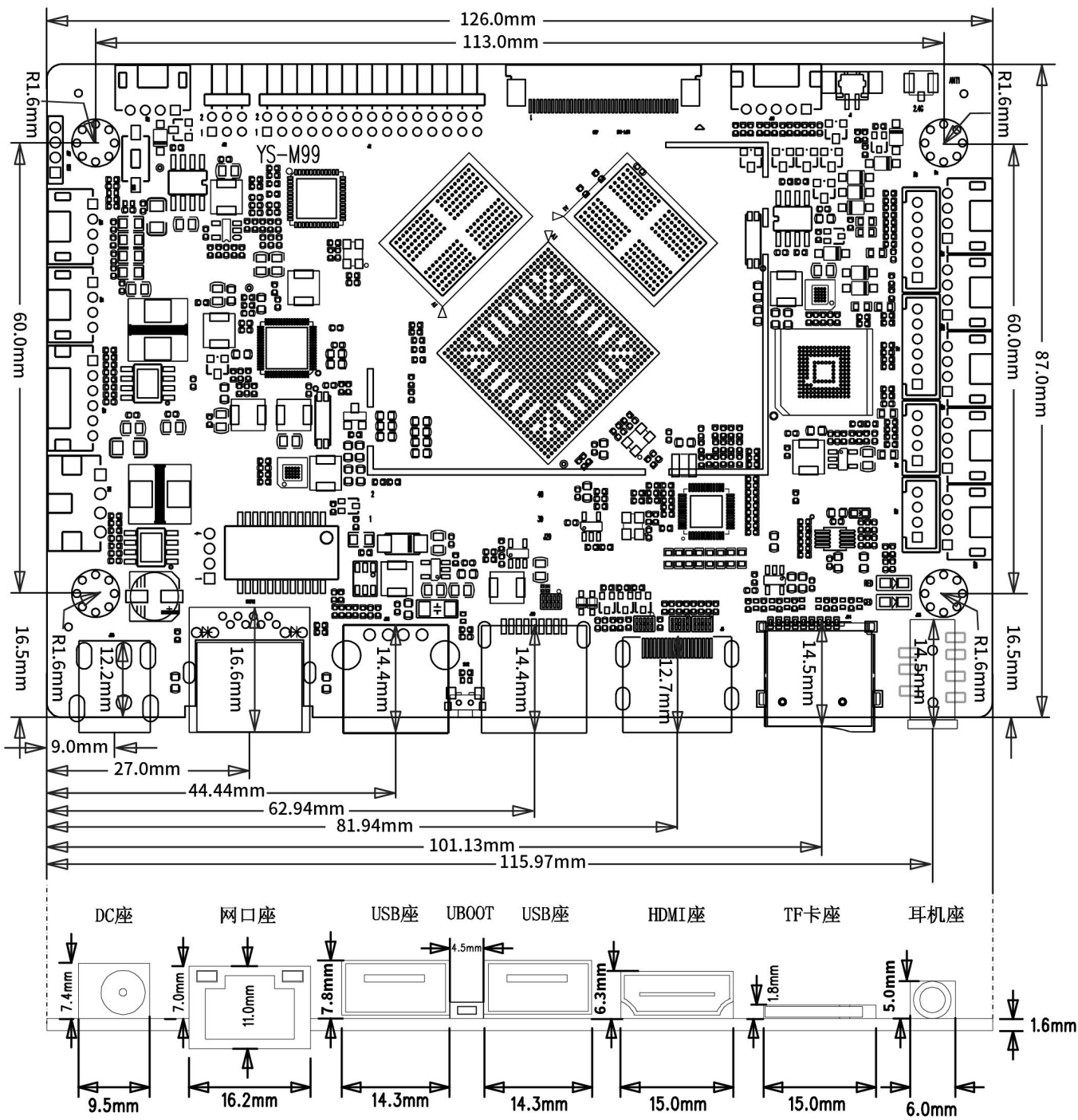
尺寸图
