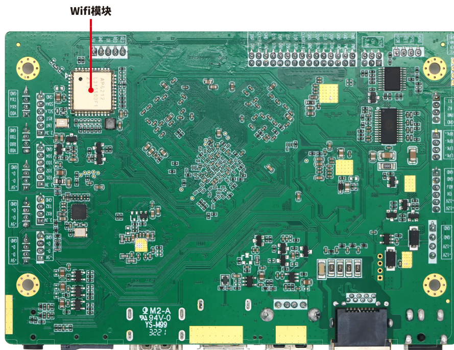
背面接口图
