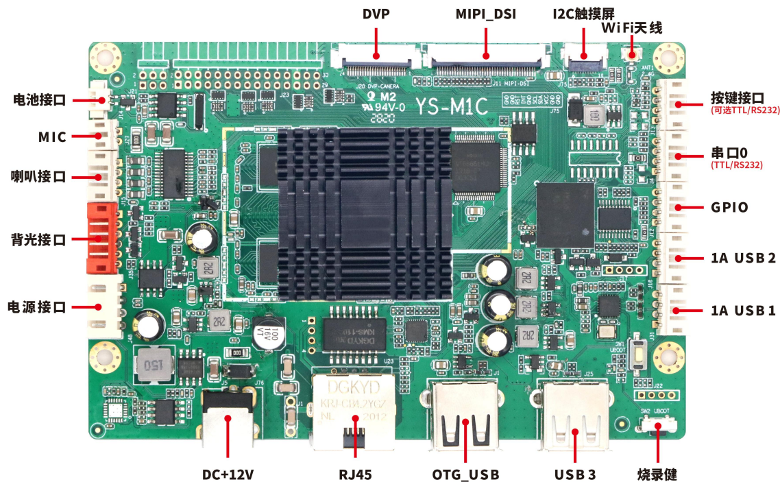
MIPI 版本正面接口图
