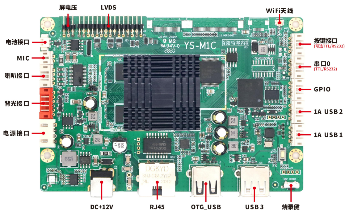
LVDS 版本正面接口图
