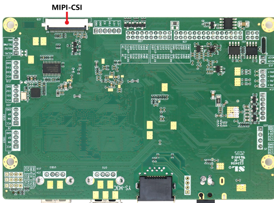
背面接口图
