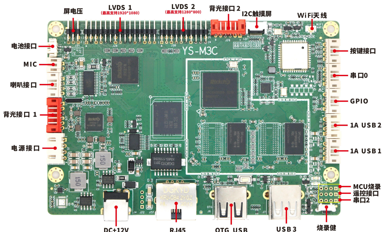
正面接口图
