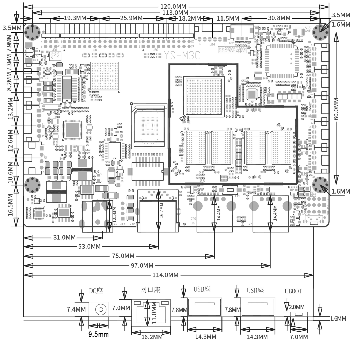
尺寸图
