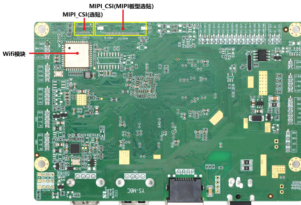
LVDS 版本背面接口图
