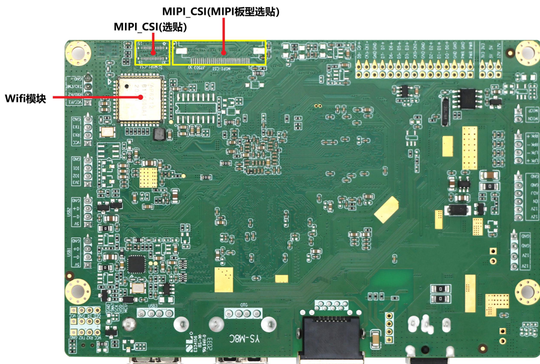
MIPI 版本背面接口图
