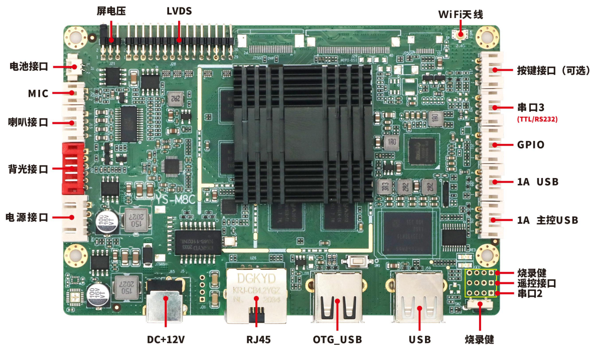
LVDS 版本正面接口图
