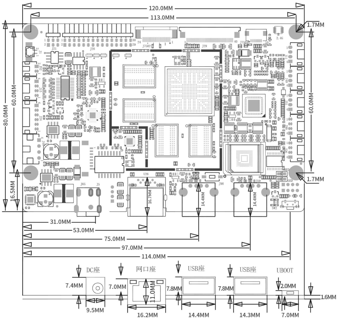
尺寸图
