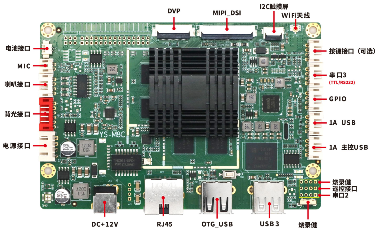
MIPI 版本正面接口图
