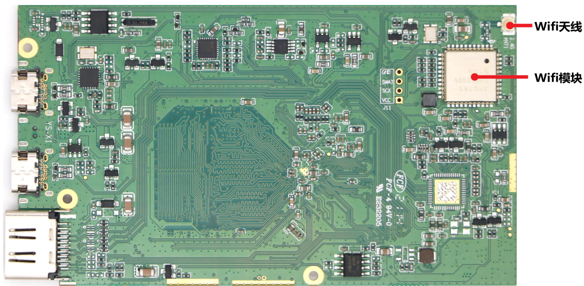
背面接口图
