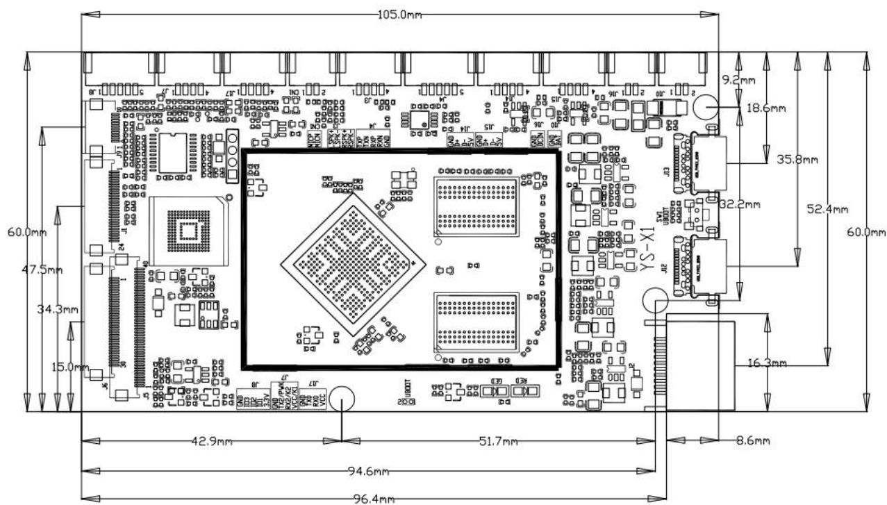
尺寸图
