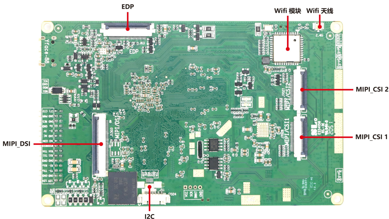
常规板背面接口图
