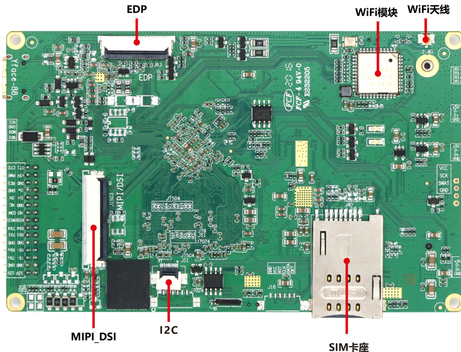
带 4G 模块背面接口图
