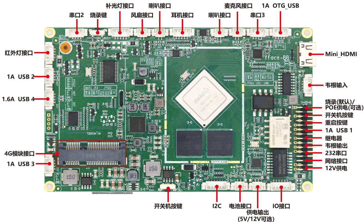
带 4G 模块正面接口图
