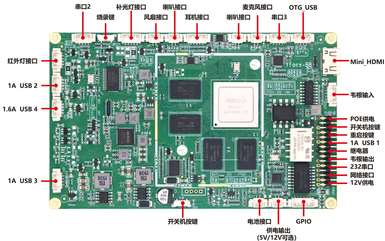
常规板正面接口图
