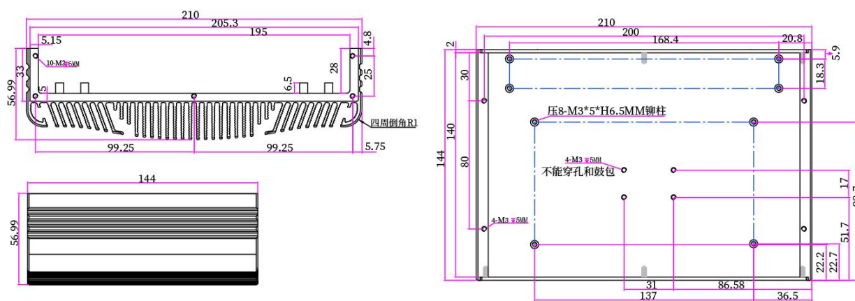
尺寸图
