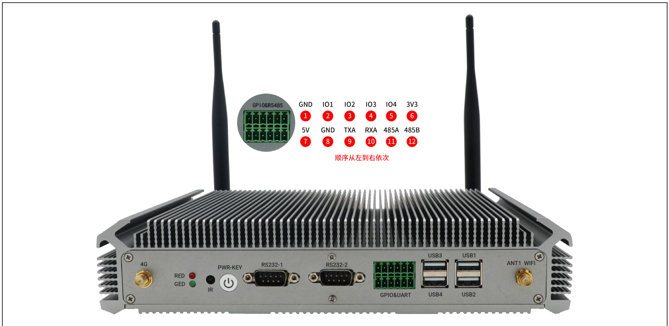
正面图
