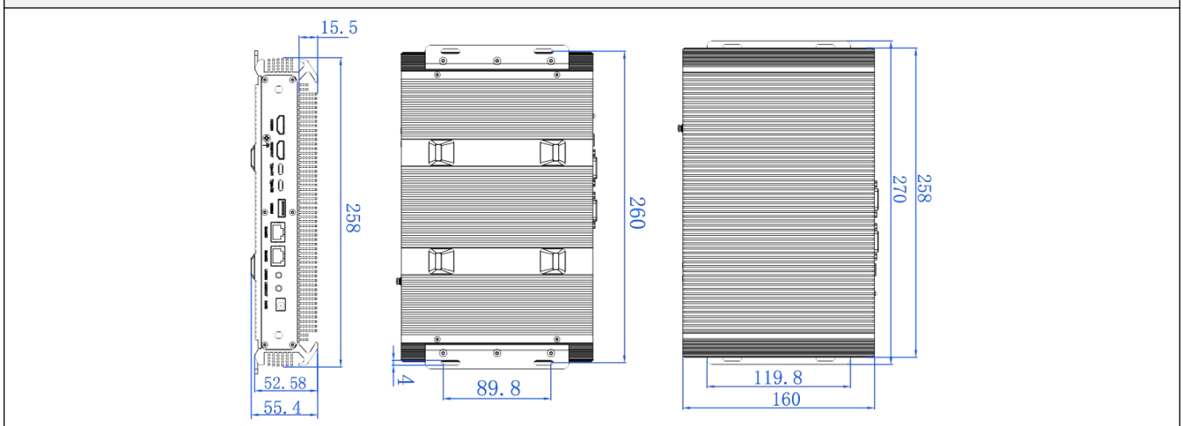
尺寸图
