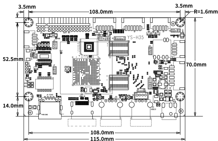
外形尺寸图
