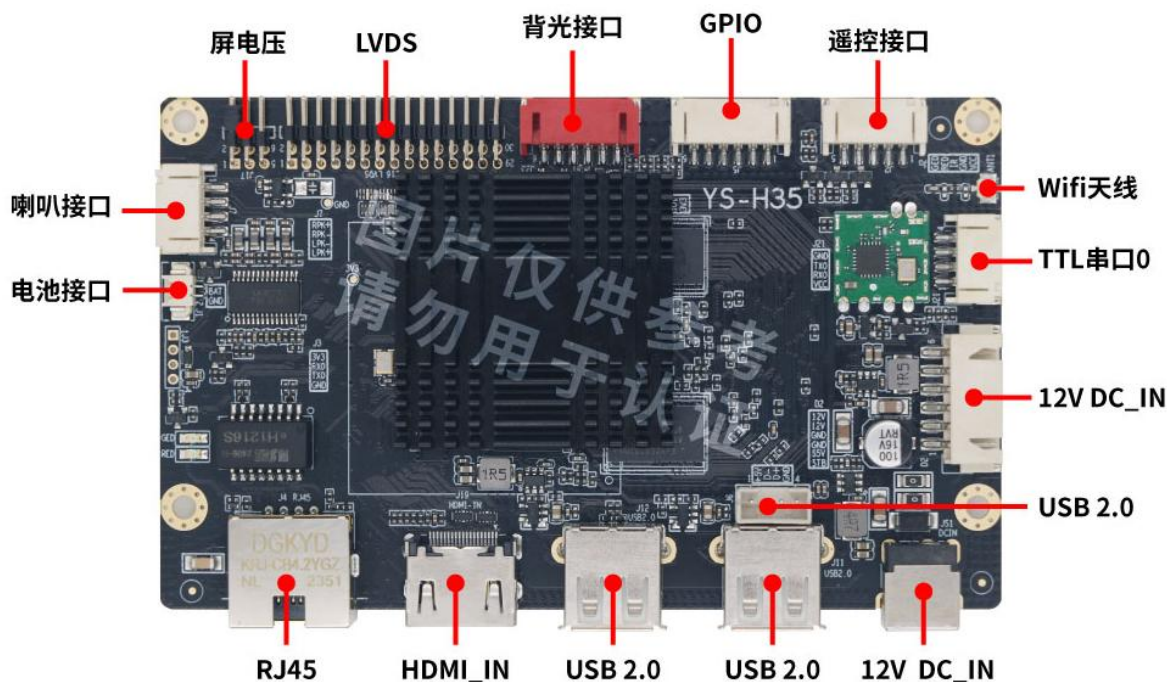
正面接口图
