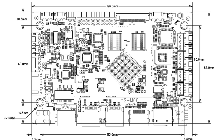
外形尺寸图
