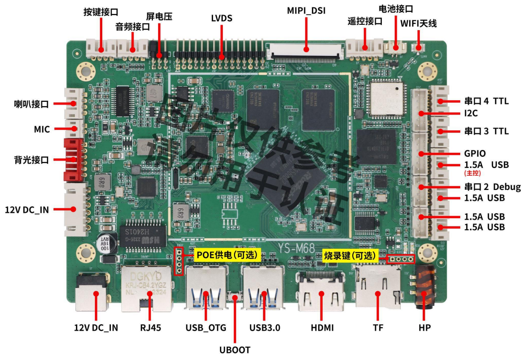
正面接口图
