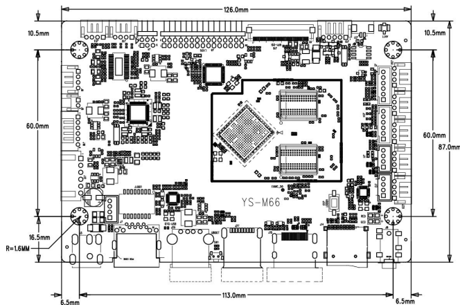
外形尺寸图
