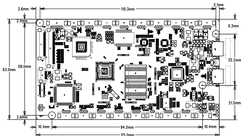
外形尺寸图
