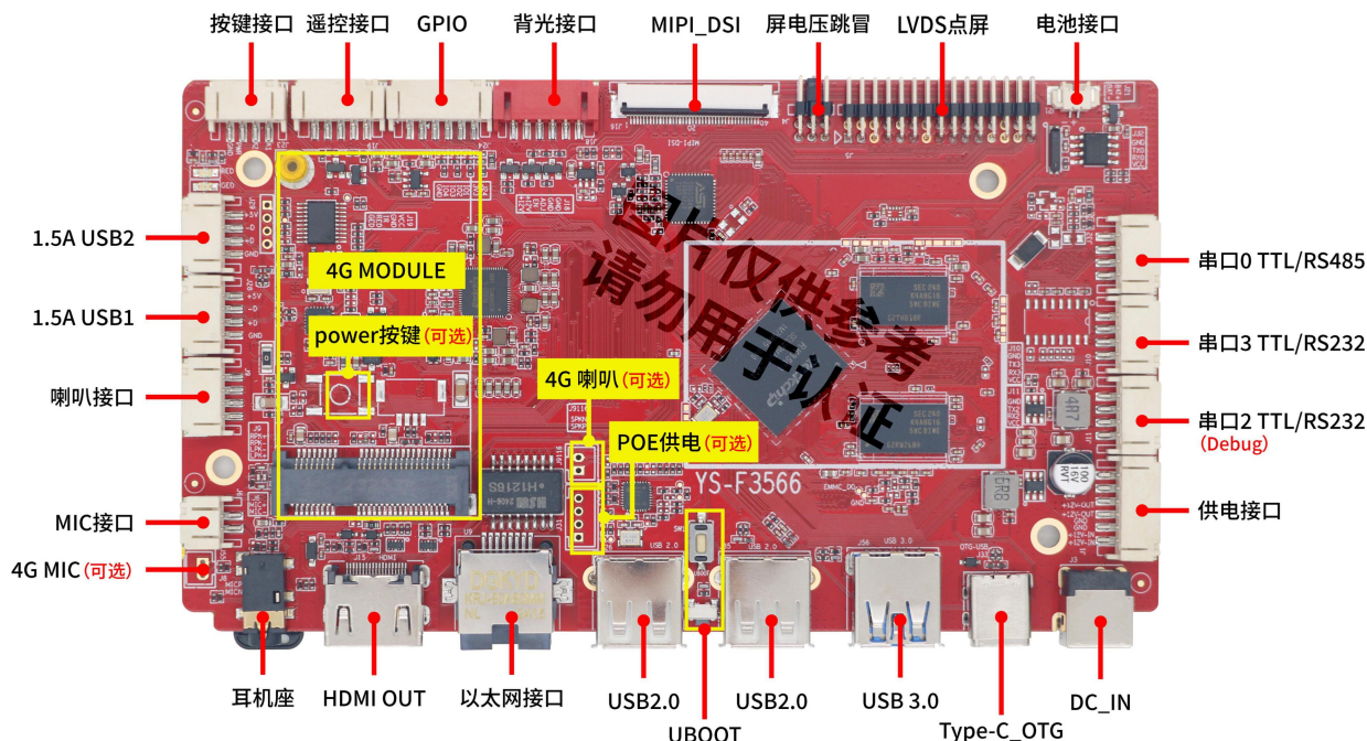
正面接口图
