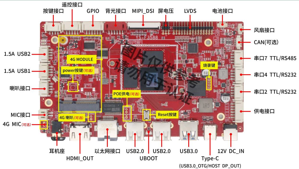
正面接口图
