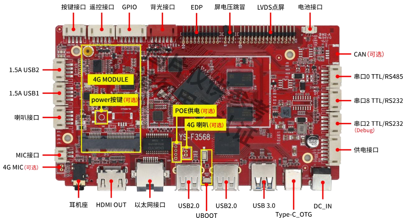
正面接口图
