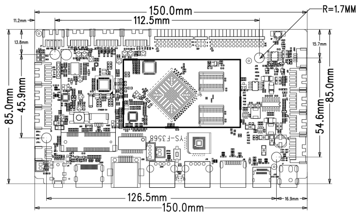
外形尺寸图
