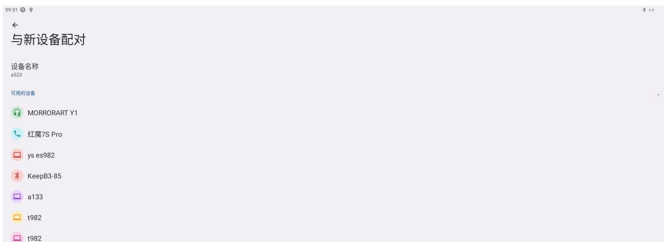
蓝牙界面
