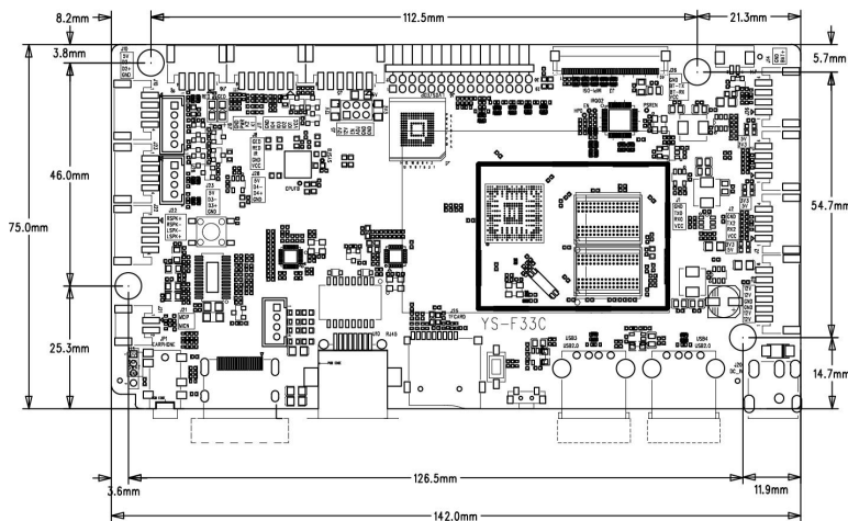
外形尺寸图
