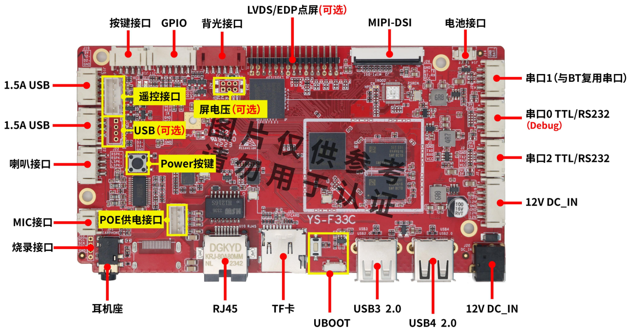
正面接口图
