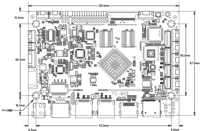
外形尺寸图
