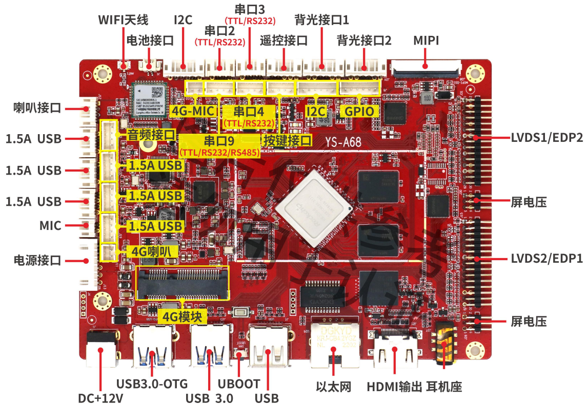
正面接口图
