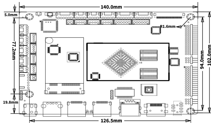
外形尺寸图
