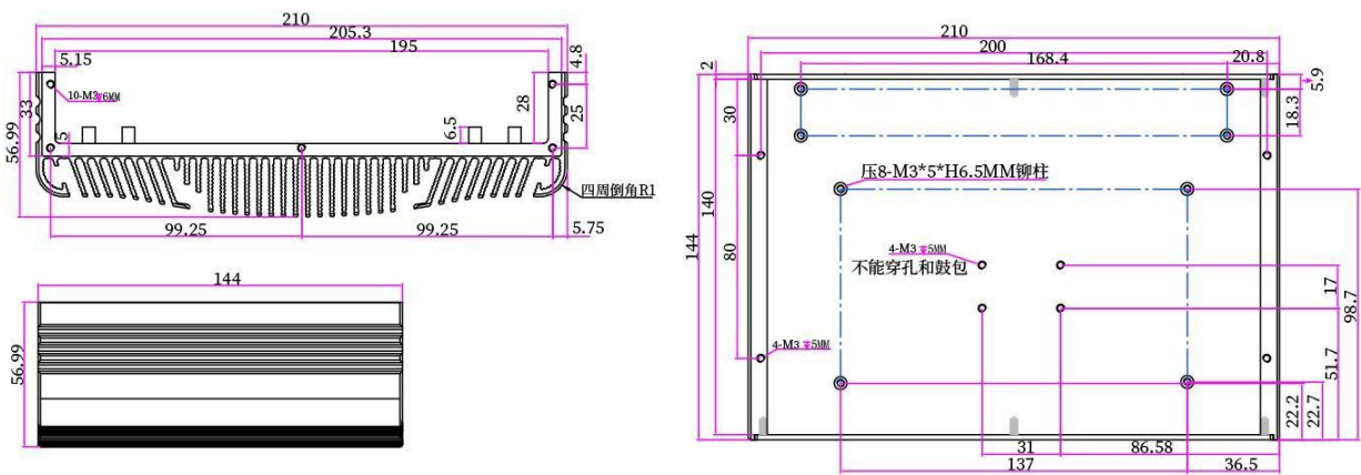
尺寸图
