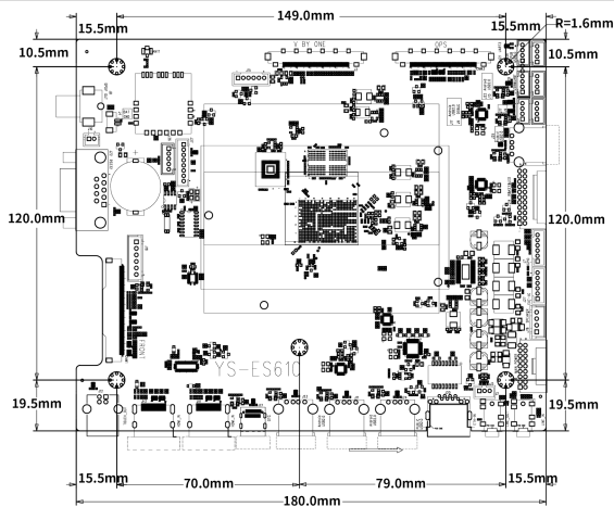
外形尺寸图
