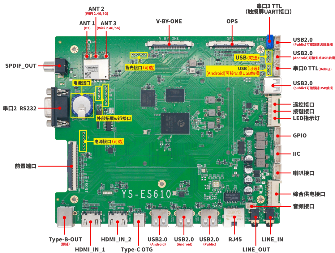
正面接口图
