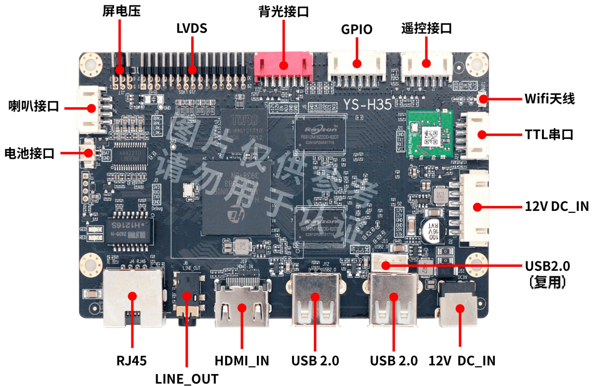
正面接口图
