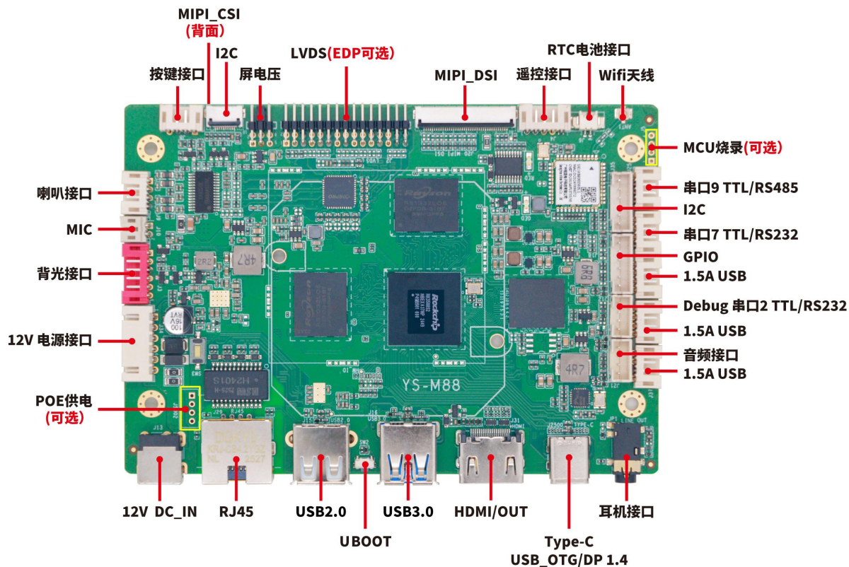
正面接口图
